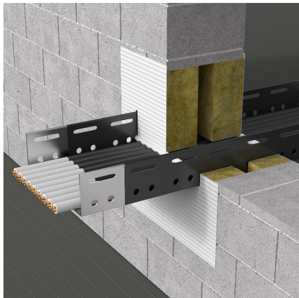
Rysunek 4.1: Zastosowanie płyty INTU FR BOARD A
