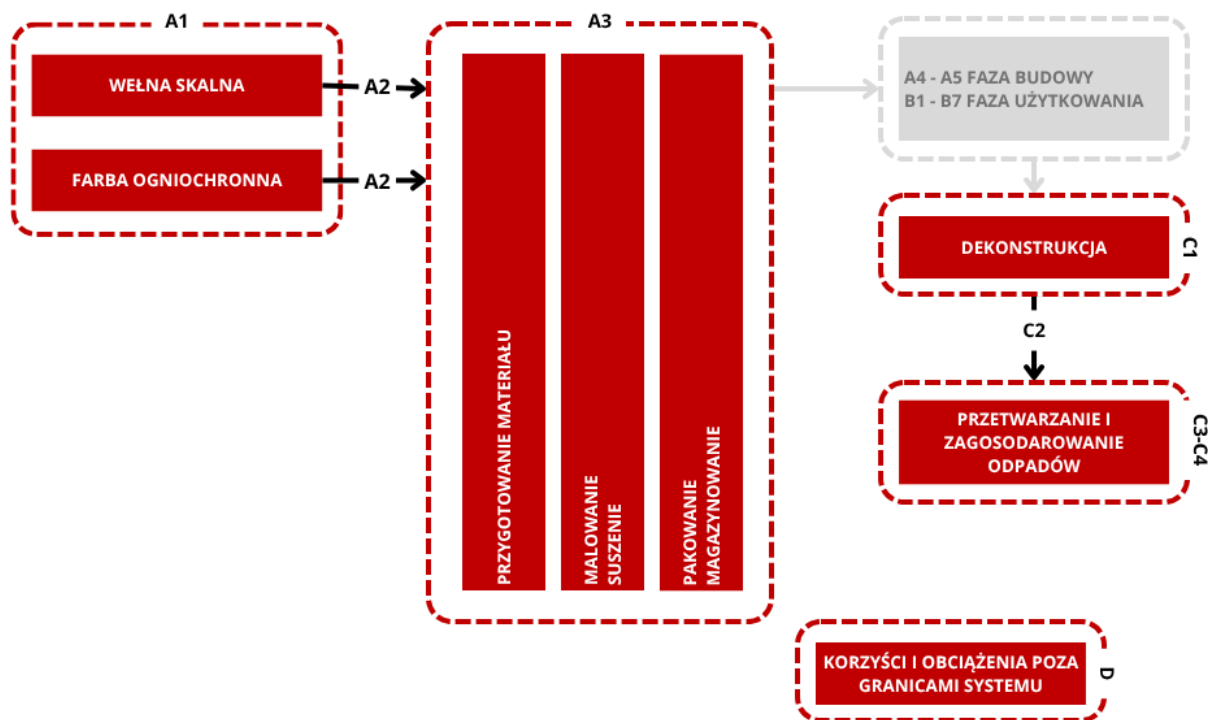
Rysunek 5.1: Granice systemu dla charakterystyki środowiskowej płyt ogniopHONNE
