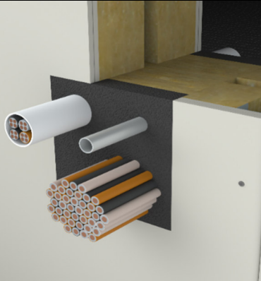
Rys.5 Uszczelnienie przejść elektrycznych / mieszanych w ścianie podatnej / sztywnej A \geq 100 mm
