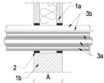
Rys.6 Uszczelnienie przejść wiązek mieszanych w ścianie podatnej / sztywnej A \geq 100 mm
